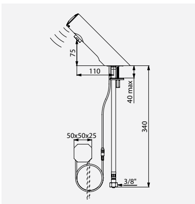
TEMPOMATIC 4 elektronische kraan op netspanning DELABIE ref.: 440100
