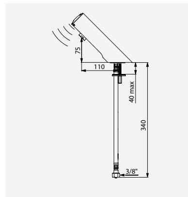
TEMPOMATIC 4 elektronische kraan op batterijen DELABIE ref.: 440106
