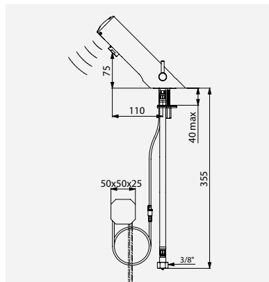
TEMPOMATIC 4 elektronische mengkraan op netspanning DELABIE ref.: 490100
