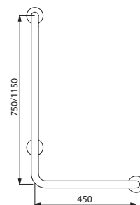
Rechts model 5070D/5071D
