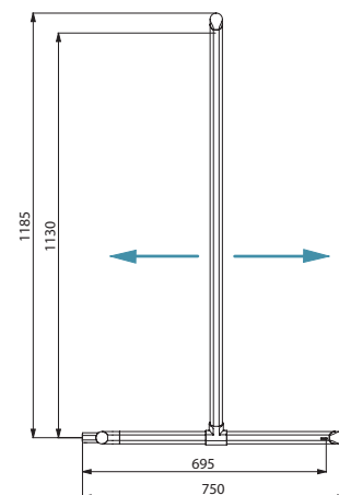
Plaatsing van de verticale stang regelbaar links of rechts
