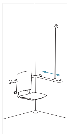
Plaatsing van de verticale stang regelbaar links of rechts (ref. 5481N)
