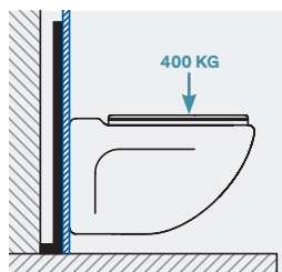
TEMPOFIX 3 zelfdragend
