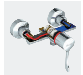
Lichaam met gladde binnenkant
